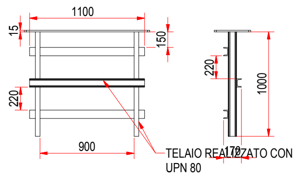
CONTROPIASTRA E TELAIO
