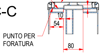
TUB 20X20 SP.3 FISSAGGIO PROFILO
