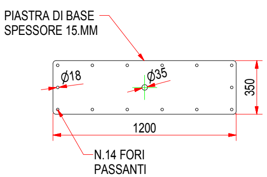
PIASTRA DI BASE : ALU 059
